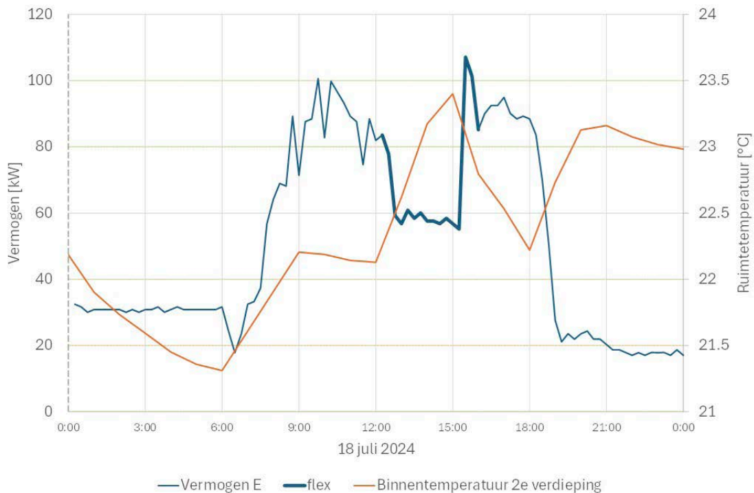
Figuur 1: Afname elektriciteit en binnentemperatuur (kantoren Veolia) bij experiment 1
