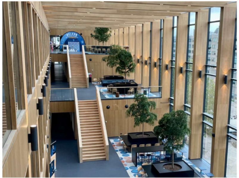
Foto 5: Het grote en hoge atrium wordt gebruikt om een groot deel van de toegevoerde lucht retour te halen.
