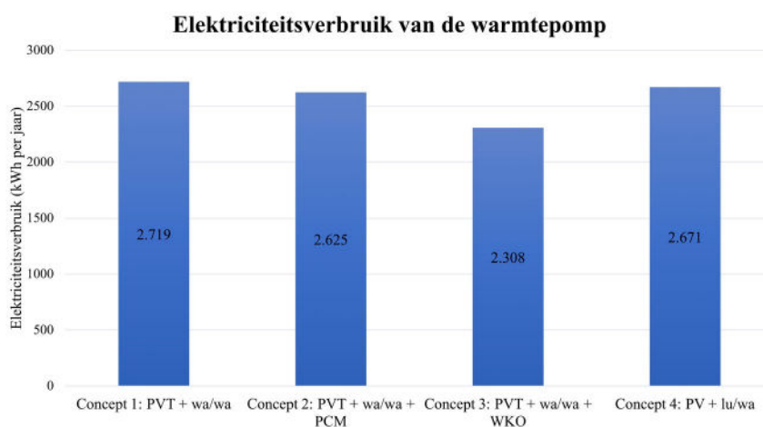
Figuur 5: Elektriciteitsverbruik van de warmtepomp per concept.
