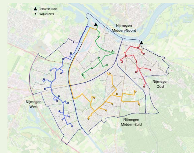
Figuur 3: Mogelijke routes van hoofdtransportleidingen voor warmtenetten in Nijmegen in het geval van aquathermie.
