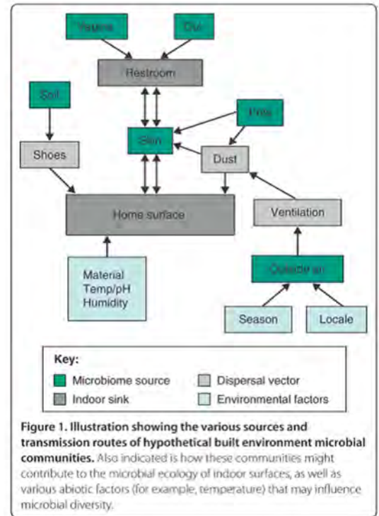
-Figuur 12- Bronnen en transmissies van micro-organismen
