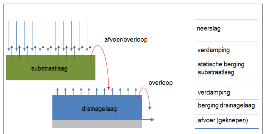
-Figuur 1- Modellschematisering van een groen(blauw) dak met substraatlaag (groen) en daaronder de drainagelaag (blauw)
