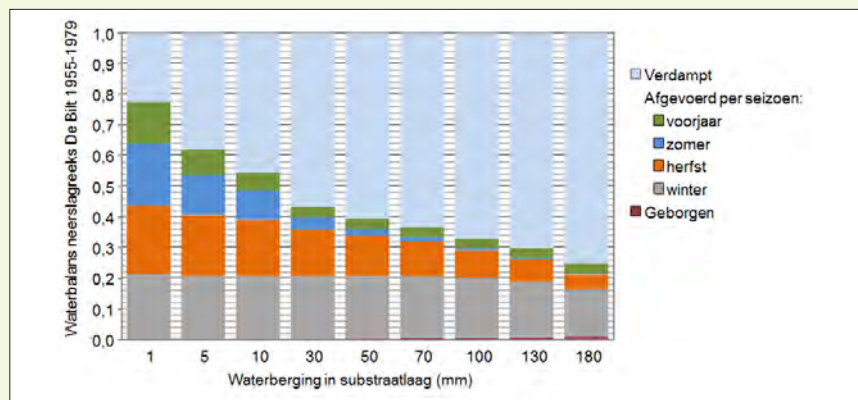
-Figuur 2- Waterbalans van 25 jaar neerslag op een groen dak, voor verschillende waterberging in de substraatlaag
