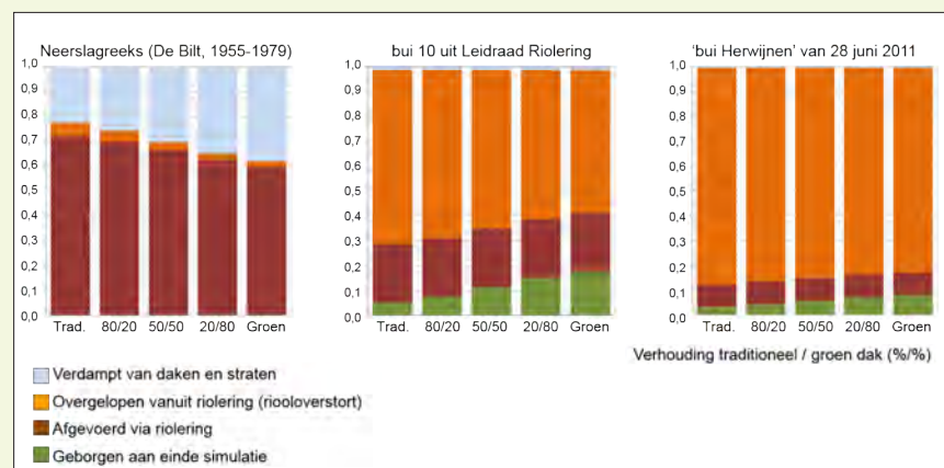
-Figuur 4- Waterbalans van 25 jaar neerslag (links), bui 10 (midden) en 'bui Herwijnen' (rechts) op een wijk, voor verschillende verhoudingen van traditionele/groenblauwe daken
