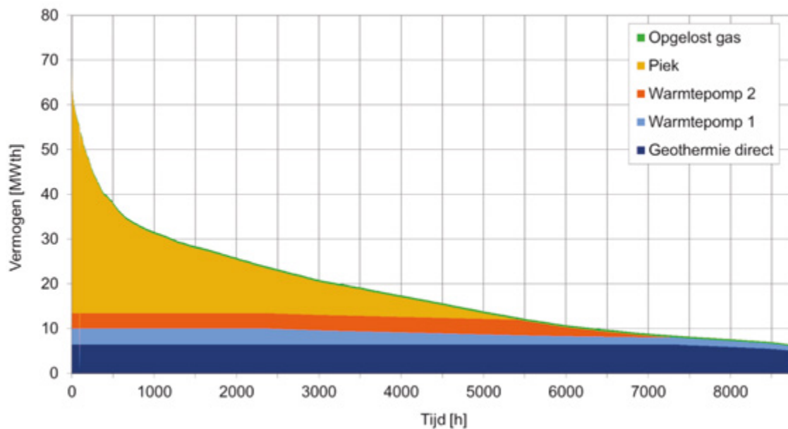
Figuur 2: Jaarbelasting duurkromme van een warmtenet met een piekvraag van 60 MWt en een geothermie project met een debiet van 215 m 3 /uur bij een productie temperatuur van 80°C. Nettemperatuur is 100°C aanvoer en 50°C retour.
