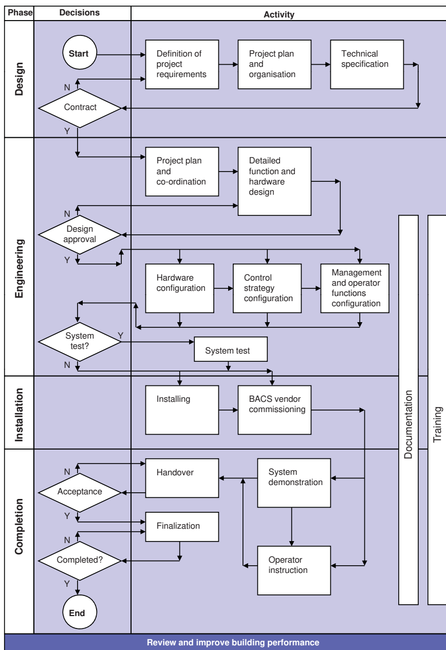
Mogelijke opeenvolging van beslissingsmomenten en acties per fase van het implementatieproces van een gebouwbeheersysteem volgens NEN-EN-ISO 16484
