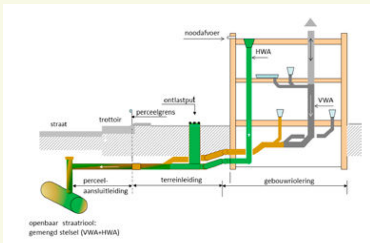
-Figuur 1- Gemengd stelsel met gezamenlijke perceelaansluiting vuilwaterafvoer (VWA) en hemelwaterafvoer (HWA)
