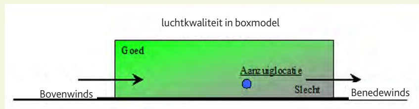
-Figuur 4- Invloed aanzuiglocatie op de luchtkwaliteit
