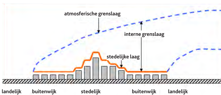
-Figuur 2- Laagvorming boven stedelijke gebieden
