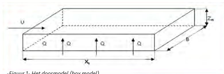
-Figuur 1- Het doosmodel (box model)
