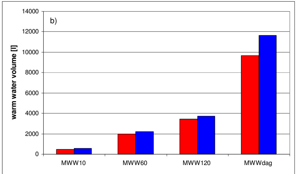
Figuur 7-2 De kentallen voor warmwaterverbruik voor hotel I (a) en hotel II (b), afgeleid uit metingen (rood) en berekend met de ontwerprekenregels (blauw). Er bestaan geen andere richtlijnen om deze kentallen te berekenen.
