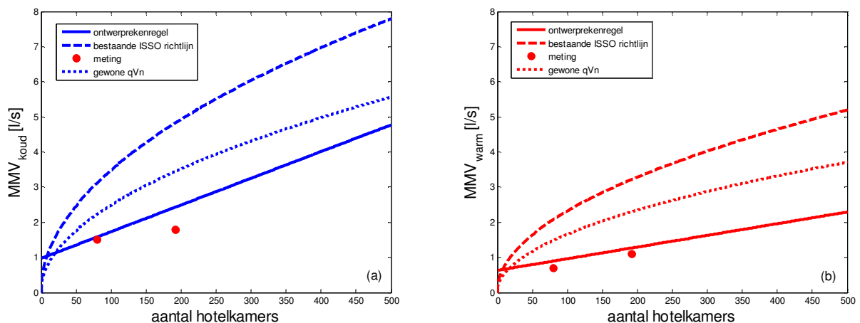
Figuur 7-1 Maximum Moment Volumestroom voor koud (a) en warm (b) water voorspeld met de SIMDEUM-ontwerprekenregel (-), de ISSO ontwerprichtlijn (- -) en de q\sqrt{n} - of q\sqrt{\Sigma TE} -methode (...) voor zakelijke hotels en vergeleken met metingen van MMV in hotel I en II (•).
