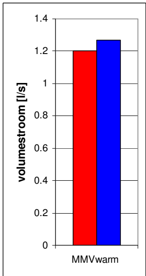
Figuur 7-2 De kentallen voor warmwaterverbruik voor hotel I (a) en hotel II (b), afgeleid uit metingen (rood) en berekend met de ontwerprekenregels (blauw). Er bestaan geen andere richtlijnen om deze kentallen te berekenen.
