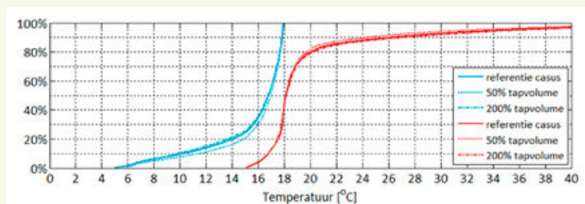
-Figuur 4- Cumulatieve frequentieverdeling voorkomende temperaturen bij verschillende tapvolumes. De rode lijnen representeren de warmtapwaterleidingen, de blauwe de koud tapwaterleidingen.
