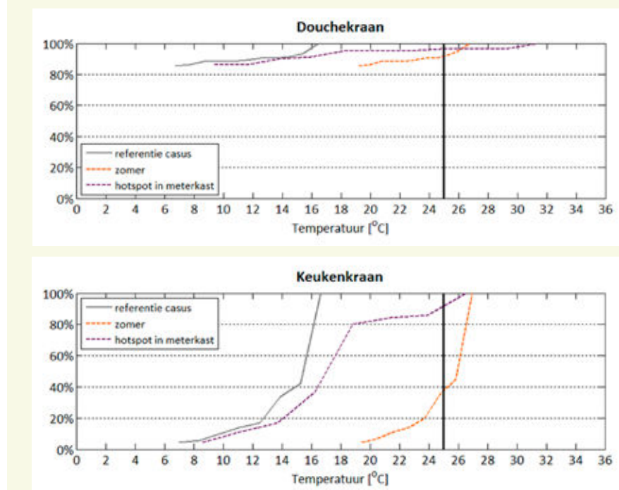
-Figuur 3- Cumulatieve frequentieverdeling van de koudwatertemperatuur tijdens verbruik voor verschillende situaties waarbij het water temperaturen bereikt boven de 25°C.
