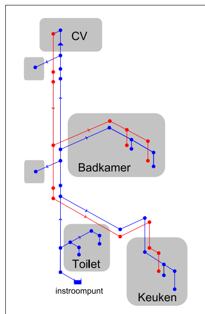
-Figuur 1- Schematische weergave model woninginstallatie. Blauwe lijnen zijn drinkwaterleidingen, rode lijnen zijn warmtapwaterleidingen. Het instroompunt bevindt zich onderaan in de figuur. De tappenpunten (uitstroompunten) zijn omgeven door grijze vlakken. De pijlen geven de stroomrichting aan.
