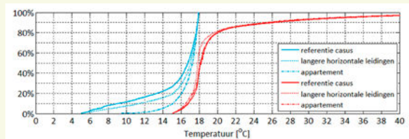
-Figuur 5- Cumulatieve frequentieverdeling voorkomende temperaturen in verschillende woningtypen. De rode lijnen representeren de warmtapwaterleidingen, de blauwe de koudtapwaterleidingen.
