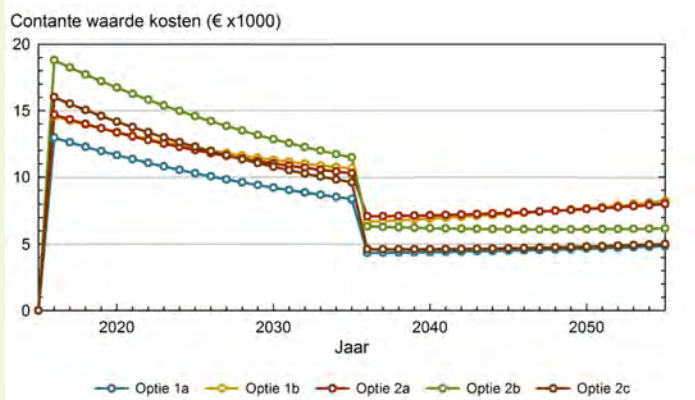
-Figuur 3- Verloop contante kosten warmtapwatersystemen
